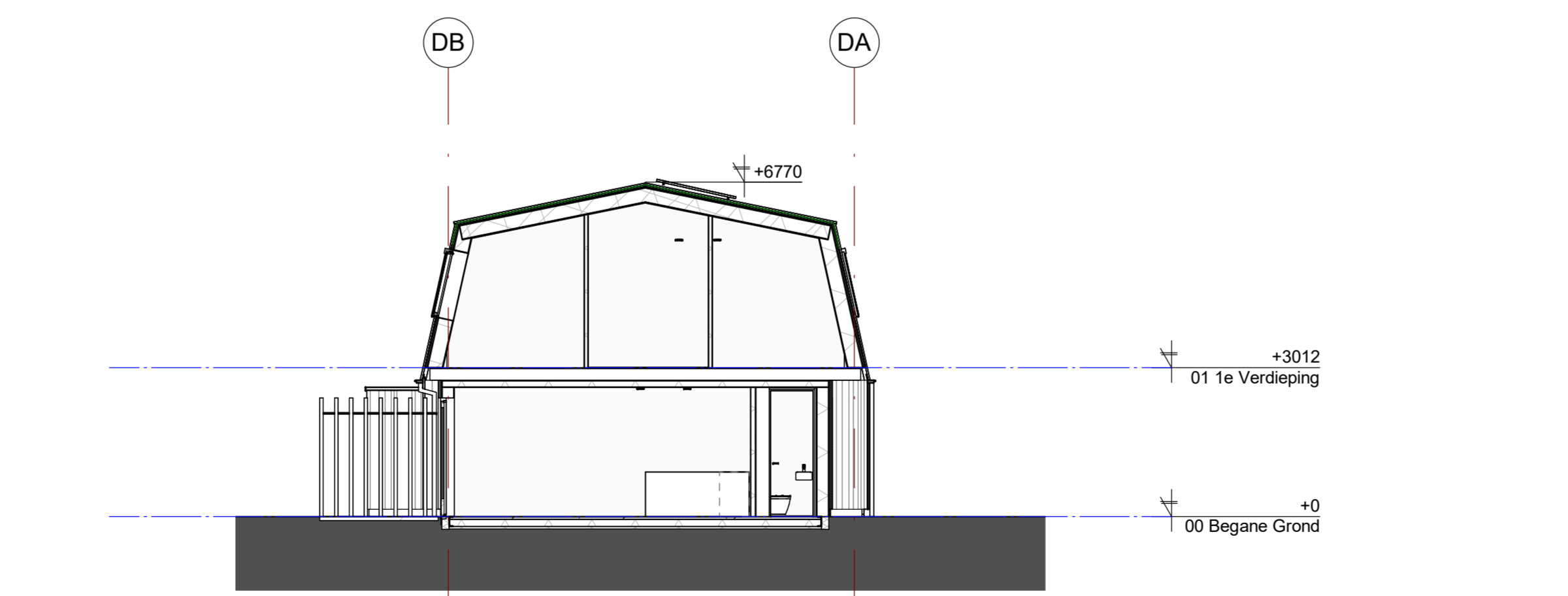
Doorsnede D2
