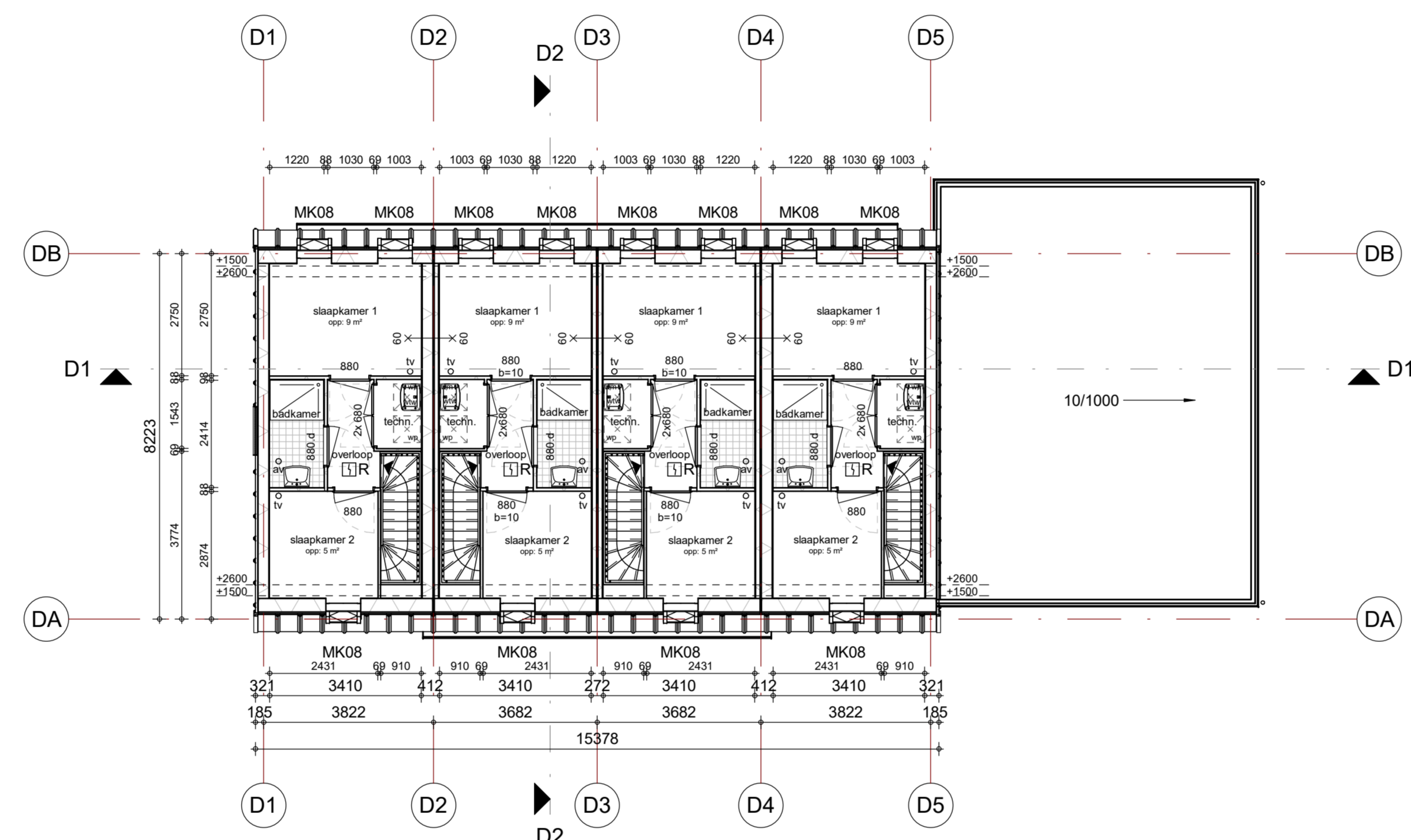
1e Verdieping
