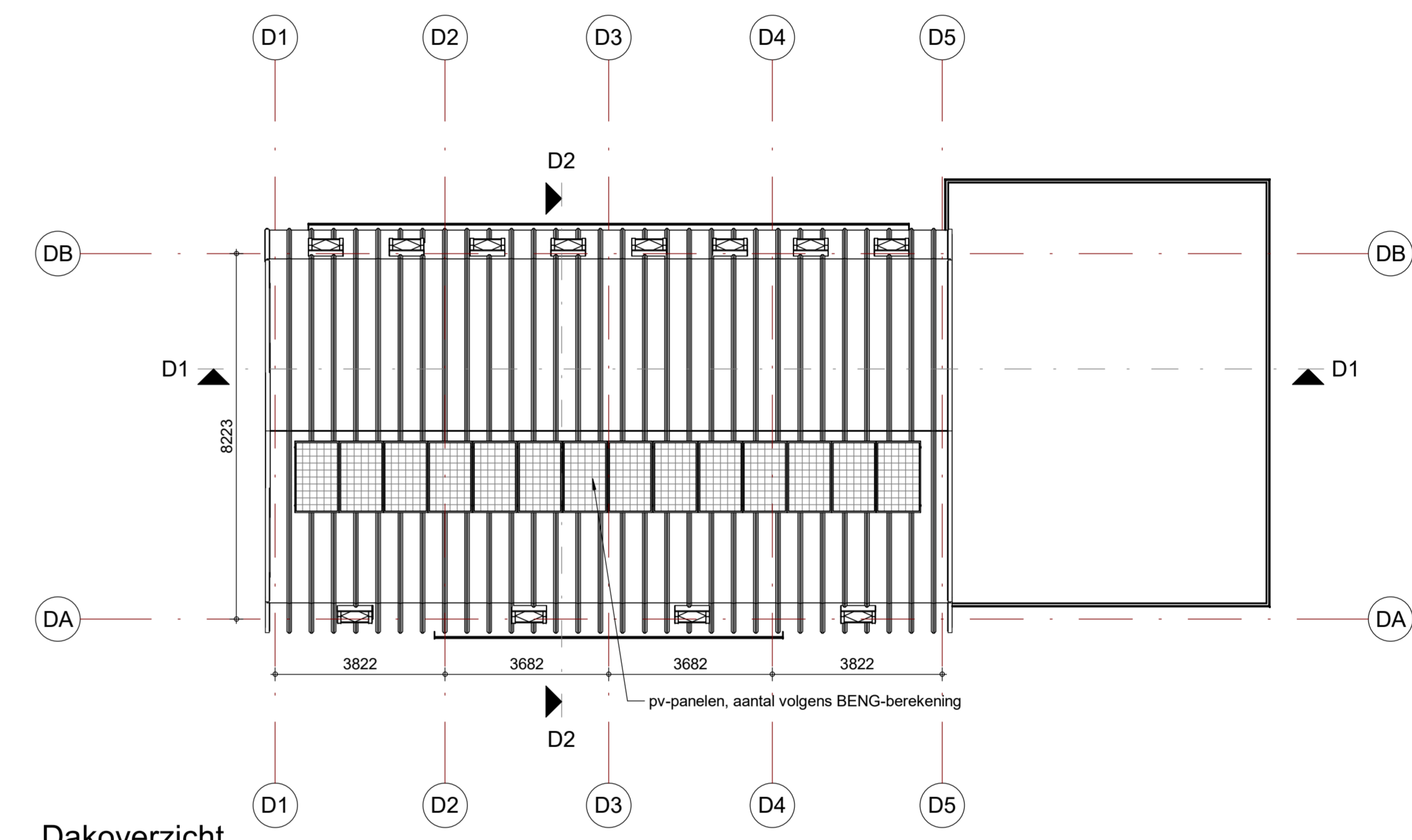
Dakoverzicht
